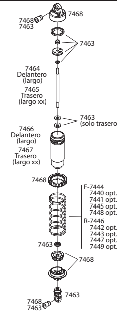
D. Instalación/extracción del pistón
